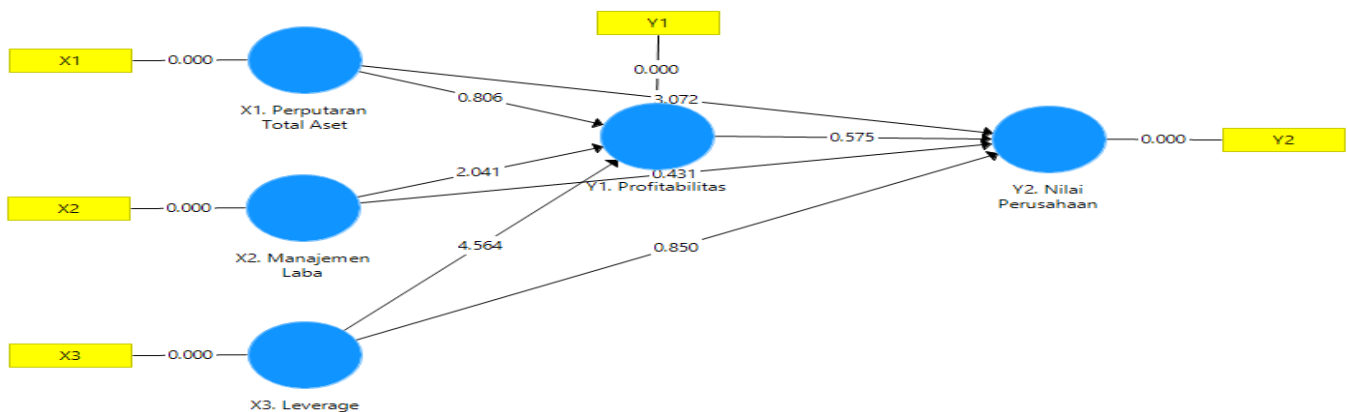
Gambar 2. Hasil Uji Model Struktural dengan Aplikasi Smart PLS
