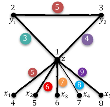
Gambar 10. Pewarnaan lokal sisi antimagic pada Squid Graph ( Sq_5 )
