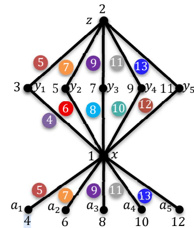
Gambar 13. Pewarnaan lokal sisi antimagic pada Jellyfish Graph (Jf_5)
