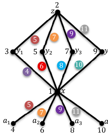
Gambar 12. Pewarnaan lokal sisi antimagic pada Jellyfish Graph (Jf_4)
