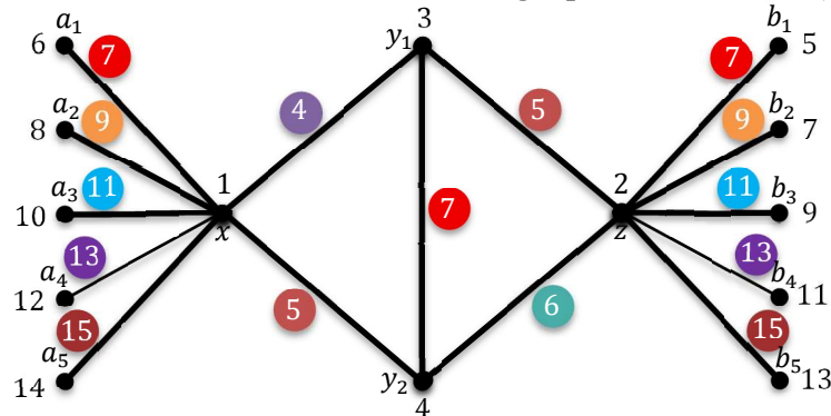
Gambar 7. Pewarnaan lokal sisi antimagic pada Crab Graph ( Cr_5 )
