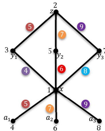
Gambar 11. Pewarnaan lokal sisi antimagic pada Jellyfish Graph (Jf_3)
