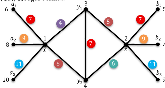
Gambar 5. Pewarnaan lokal sisi antimagic pada Crab Graph ( Cr_3 )
