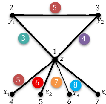
Gambar 9. Pewarnaan lokal sisi antimagic pada Squid Graph ( Sq_4 )
