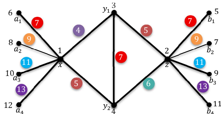
Gambar 6. Pewarnaan lokal sisi antimagic pada Crab Graph ( Cr_4 )
