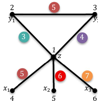
Gambar 8. Pewarnaan lokal sisi antimagic pada Squid Graph ( Sq_3 )
