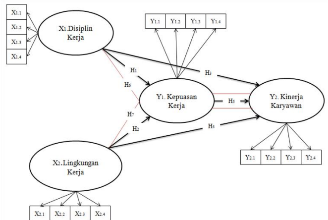
Gambar 1 Kerangka Konseptual
