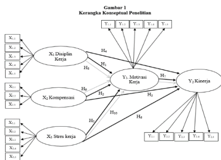
Gambar 1 Kerangka Konseptual
