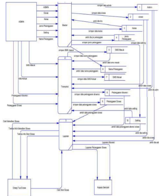
Gambar 2. DFD Level 1
