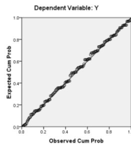
Gambar 3 Hasil Pengujian Normalitas
