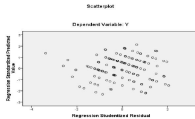
Gambar 2 Hasil Pengujian Heterokedastisitas
