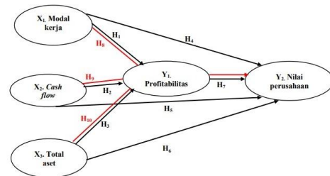
Gambar 1 Kerangka Konseptual
