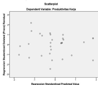
Gambar 2 Uji Heteroskedasitas
