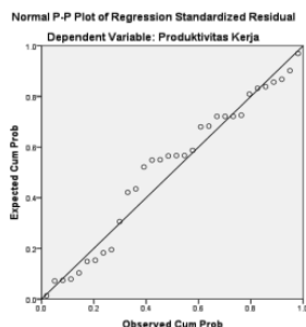
Gambar 1 Uji Normalitas Secara Grafik
