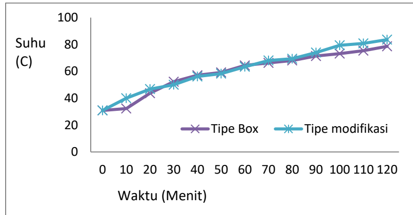
Gambar 3. Kinerja kompor surya tipe box dan tipe modifikasi dalam pemanasan air.
