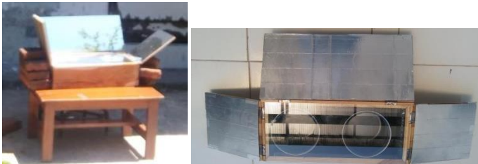
Gambar 1. Kompor surya tipe kotak ( box type )
