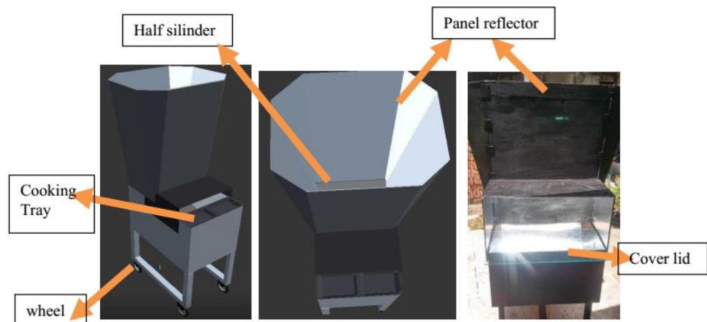
Gambar 2. Kompor surya modifikasi
