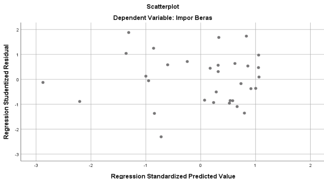
Gambar 2. Hasil Uji Heterokedastisitas (Scatterplot)
